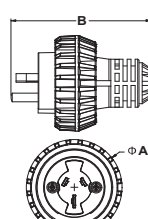
Phích Cắm Plug IP66 P-315
